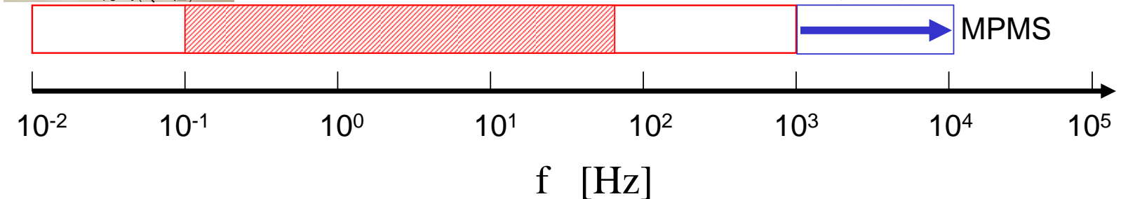
図. 我々の自作LTS-dc-SQUIDシステムとMPMS, PPMSの性能比較
